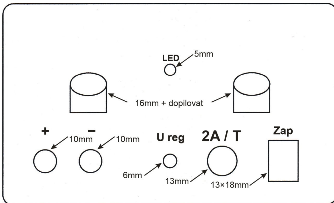
Obr. 1 přední panel
