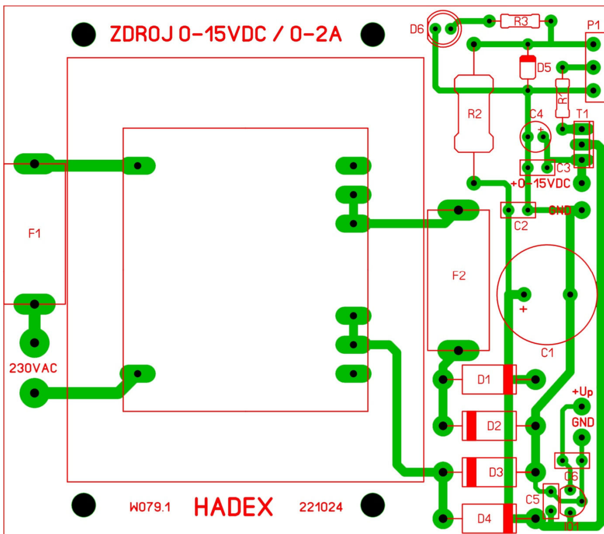
Obr. 4 osazovací plán
